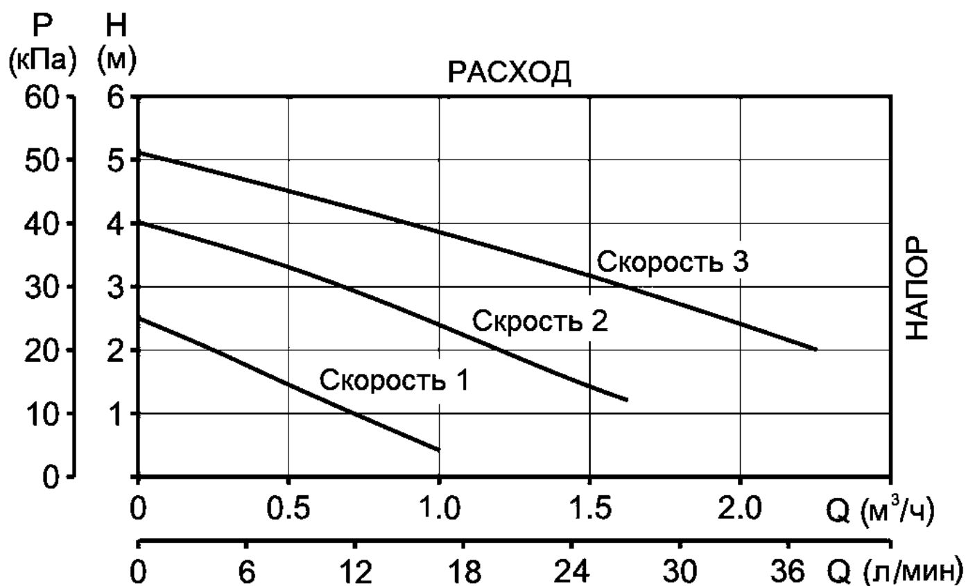
Рис. 17 Напорно-расходные кривые циркуляционного насоса электрокотла. Потери напора циркуляционного насоса «ARDERIA»
