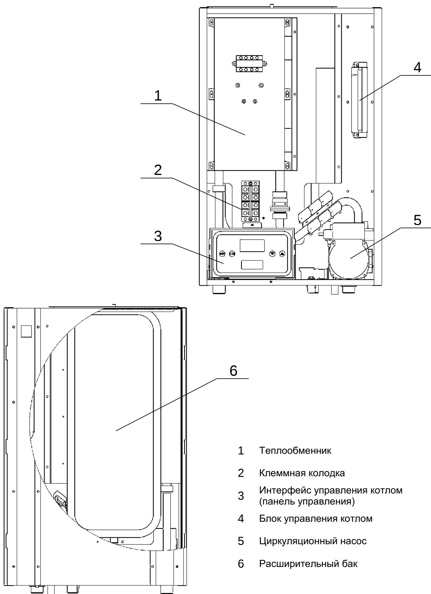
Рис. 2 Внутренне устройство
