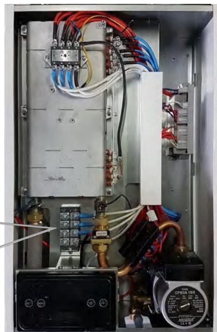
Рис. 12 Трёхфазное подключение
